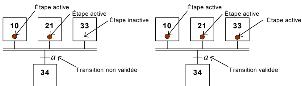
Exemple avec GRAFCET à séquences simultanées
