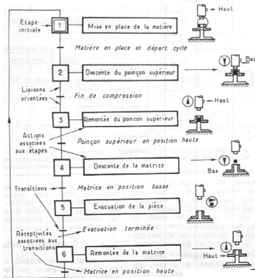
Figure 4-1 : GRAFCET de niveau 1 – Fonctionnement décrit de façon littérale
