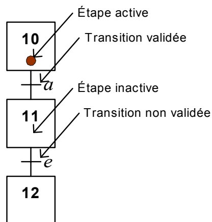
Exemple avec GRAFCET à séquence unique
